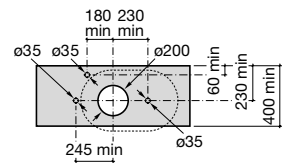
32722G..0 630 x 420 Con orificio para grifería. Pierced taphole. Trou percé pour la robinetterie. С отверстием под смеситель.
