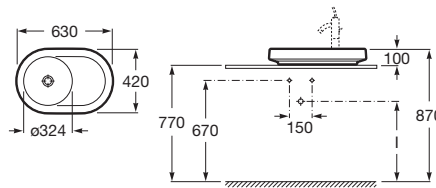
32722G..0 630 x 420 Con orificio para grifería. Pierced taphole. Trou percé pour la robinetterie. С отверстием под смеситель.
