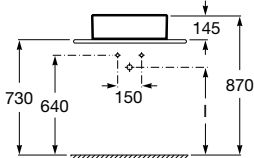
Griferia repisa
